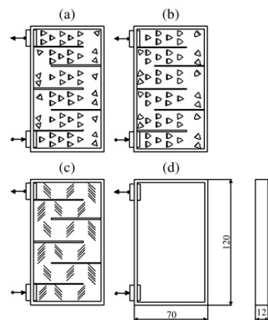
รูปที่ 12 ตัวเก็บรังสีแบบไม่มีและมีอุปกรณ์กีดขวางการไหลแบบต่าง ๆ [13]
