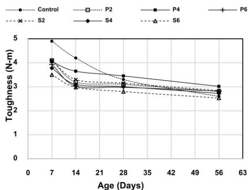
รูปที่ 14 การเปรียบเทียบความเหนียวของแผ่นคอนกรีตเสริมเส้นใยแก้ว
