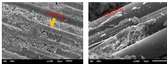
รูปที่ 15 ภาพถ่ายของตัวอย่างควบคุม (บ่มน้ำ 56 วัน)
