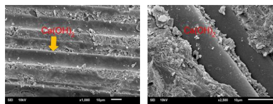
รูปที่ 16 ภาพถ่ายของตัวอย่างที่ใช้ยางพาราธรรมชาติ ร้อยละ 2 (บ่มน้ำ 56 วัน)
