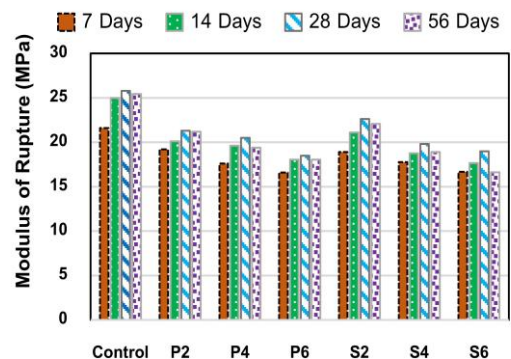
รูปที่ 11 การเปรียบเทียบหน่วยแรงดัดที่ MOR
