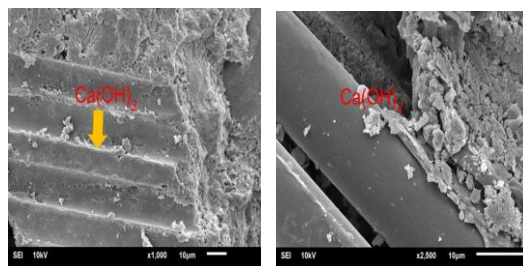
รูปที่ 17 ภาพถ่ายของตัวอย่างที่ใช้ยางพาราสังเคราะห์ ร้อยละ 2 (บ่มน้ำ 56 วัน)
