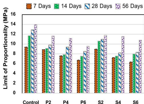
รูปที่ 10 การเปรียบเทียบหน่วยแรงดัดที่ LOP
