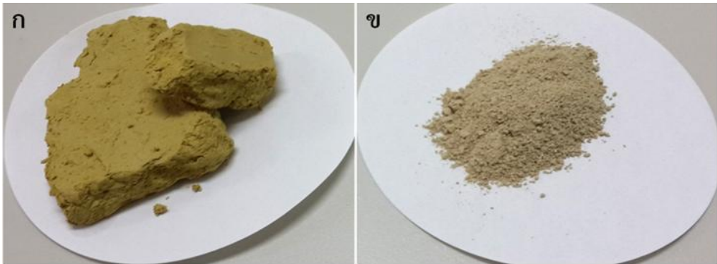
รูปที่ 1 (ก) จาโรไซต์ที่เกิดขึ้นจากโรงงานผลิตสังกะสี (ข) จาโรไซต์ที่ผ่านการอบแห้งและร่อนด้วยตะแกรง
