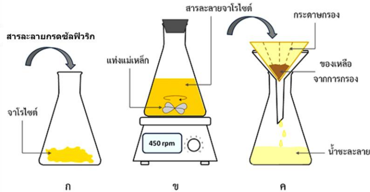
รูปที่ 2 (ก) การผสมกรดซัลฟิวริกกับจาโรไซต์ในขวดรูปชมพู่ (ข) การกวนสารละลายจาโรไซต์ด้วยเครื่องกวนระบบแม่เหล็ก (ค) การกรองสารละลายจาโรไซต์ด้วยกระดวยกรอง
