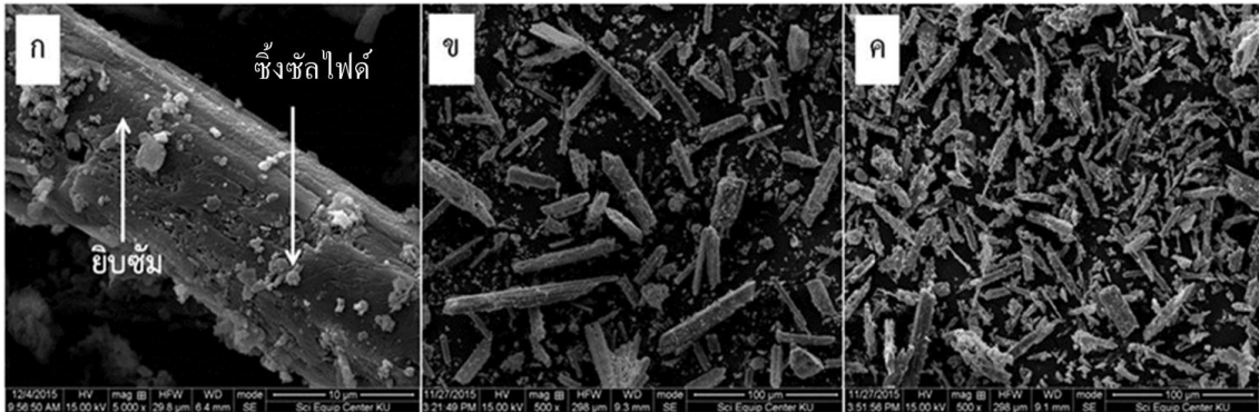
รูปที่ 4 (ก) SEM กำลังขยาย 5000X แสดงอนุภาคสังกะสีซิงค์ไฟต์บนผิวของยิบซั่ม (ข) SEM กำลังขยาย 500X แสดงลักษณะผลึกของยิบซั่มในจาโรไซท์ก่อนการชะละลาย (ค) SEM กำลังขยาย 500X แสดงลักษณะผลึกของยิบซั่มในจาโรไซท์หลังการชะละลายด้วยกรดซัลฟิวริกเป็นเวลา 24 ชั่วโมง
