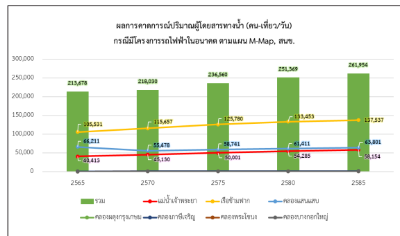
รูปที่ 6 ผลการคาดการณ์ปริมาณผู้โดยสารทางน้ำ กรณีมีโครงการรถไฟฟ้าในอนาคต ตามแผน M-Map, สนข.
