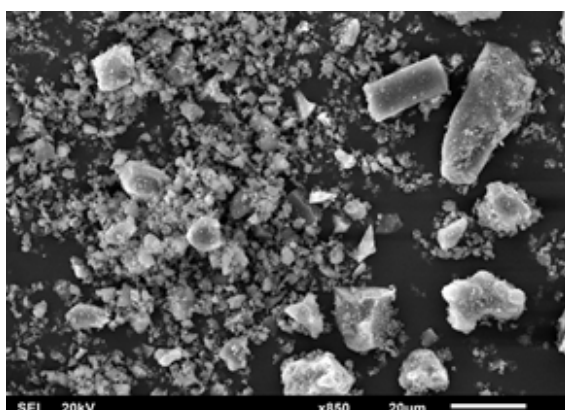
(ข) เถ้าปาล์มน้ำมันหลังบด
