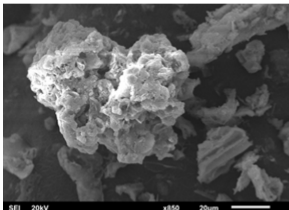
(ก) เถ้าปาล์มน้ำมันก่อนบด
