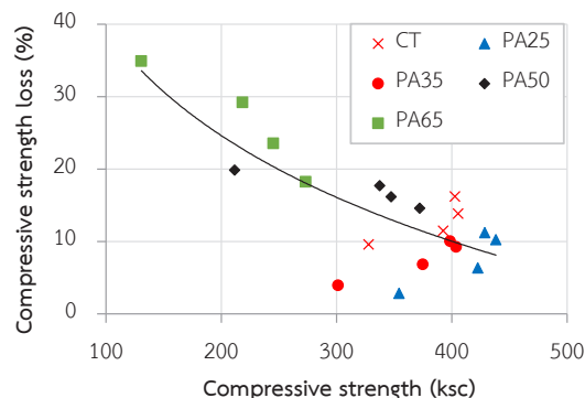
รูปที่ 7 ความสัมพันธ์ระหว่างกำลังอัดและการสูญเสียกำลังอัดของมอร์ต้าที่บ่มในน้ำพรู
