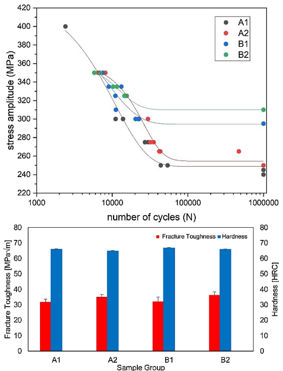
รูปที่ 11 ความต้านทานการแตกหักและความล้าของเหล็กกล้าเครื่องมือความเร็วสูง (A1 คือ M2 ที่ผ่านการอบชุบแบบดั้งเดิม, A2 คือ M2 ที่ผ่านกระบวนการโครโอเจนิคส์แบบลึกแล้วจึงตามด้วยการอบคืนตัว B1 คือ M3:2 ที่ผ่านการอบชุบแบบดั้งเดิม B2 คือ M3:2 ที่ผ่านกระบวนการโครโอเจนิคส์แบบลึกแล้วตามด้วยการอบคืนตัว) [19]
