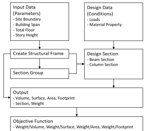
รูปที่ 2 ผังระเบียบวิธีดำเนินการประมาณน้ำหนักโครงสร้างอาคารหลักด้วยวิธีการออกแบบเชิงกำเนิด
